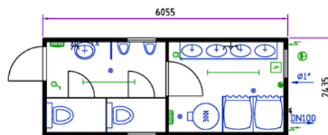
Bungalow sanitaire 20'
